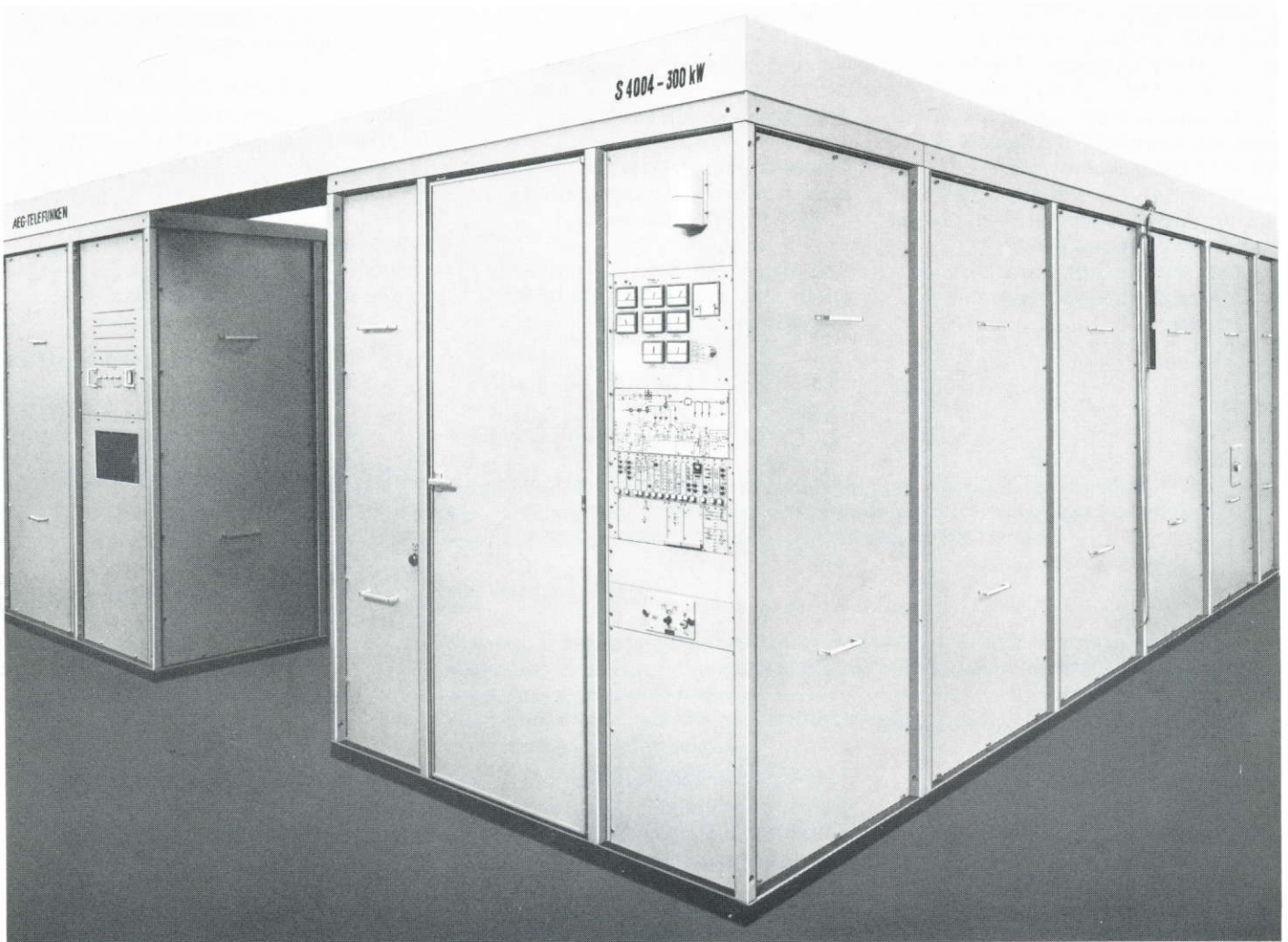
Bild 1: 300-kW-MW-Rundfunksender S 4004
