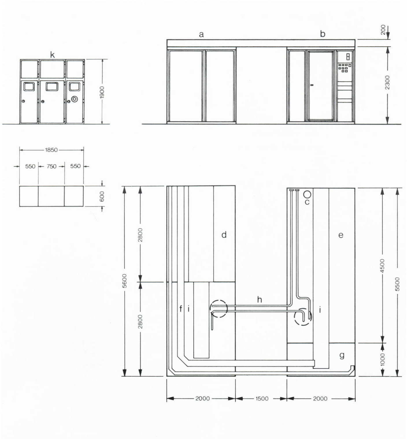
Bild 6 Maßskizze
