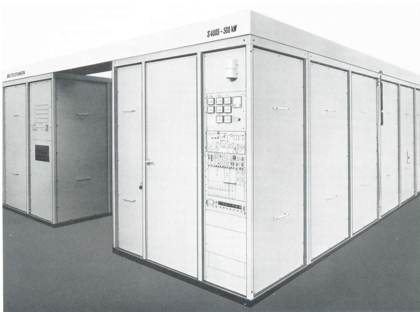
Bild 1: 500-kW-KW-Rundfunksender S 4005
