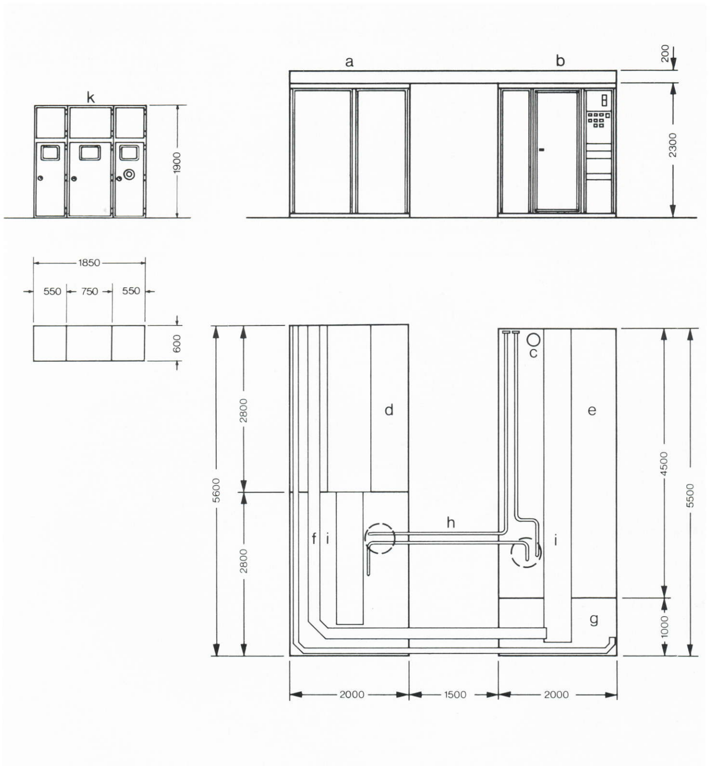
Bild 6 Maßskizze
